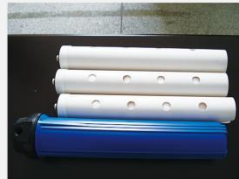
型号 : MAX-C-M31 尺寸 Size : Ø63×500mm 流量 Flow : 10-20L/min 工作压力 Working pressure : 0.1-0.4MPa
